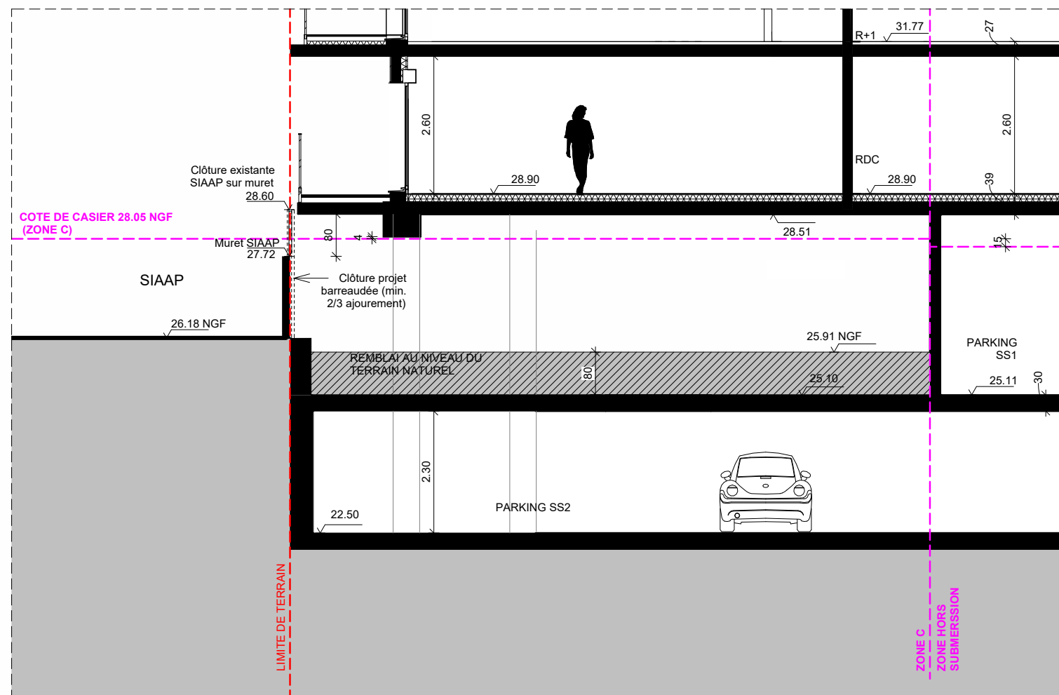
DET 4 Agrandissement du plan de coupe entre la limite SIAAP et le projet 1:100
