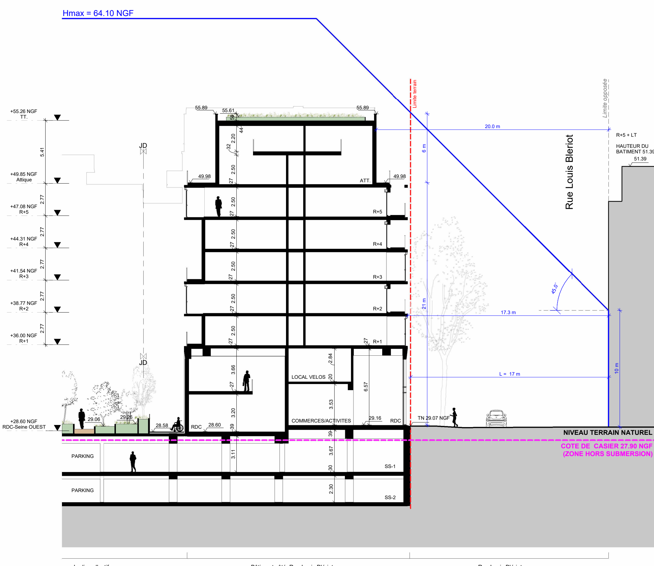
Coupe 6-6' 1:200
