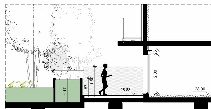
DET3 - Coupe sur terrasse privative 1:100
