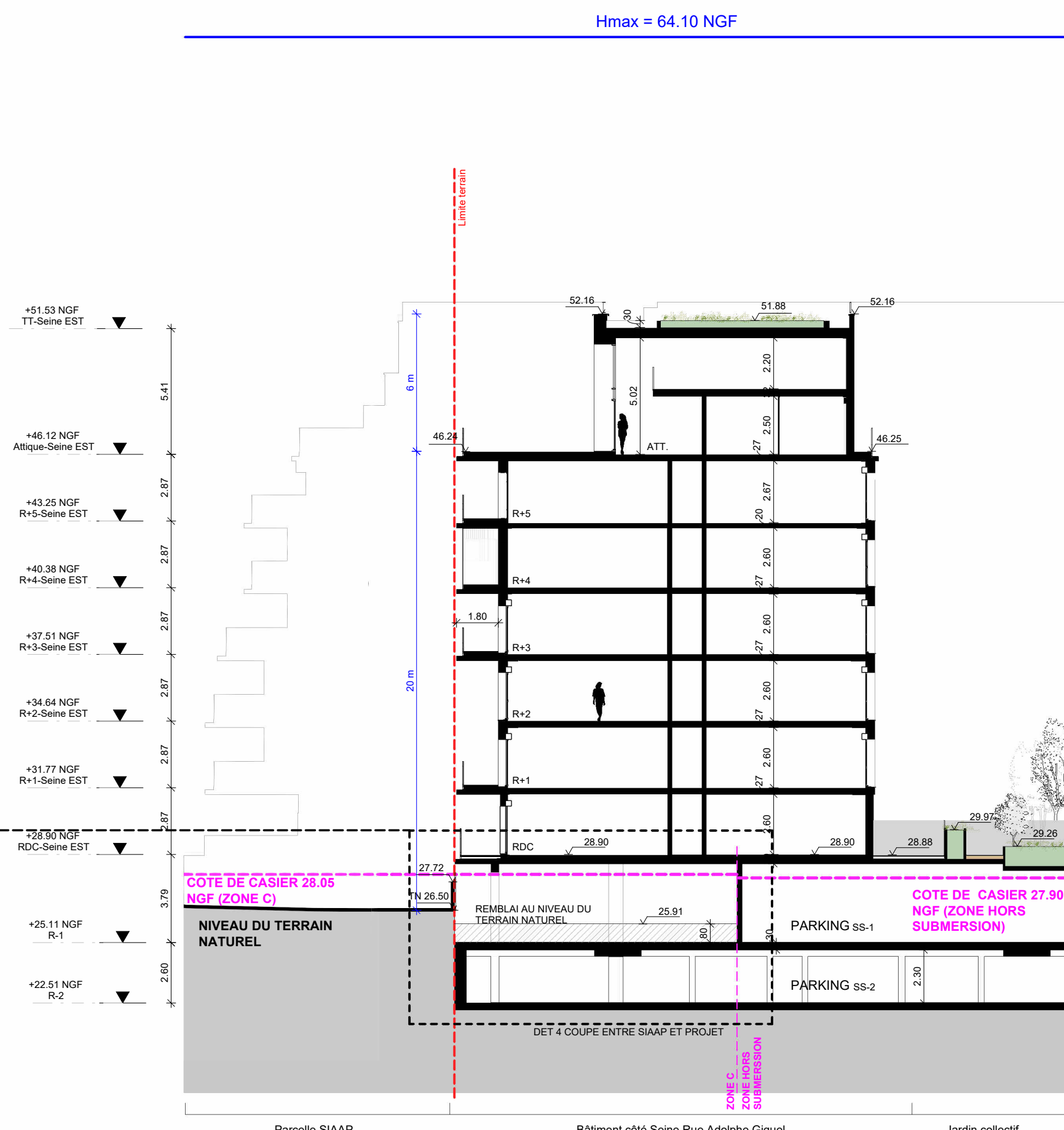
Coupe 5-5' 1:200
