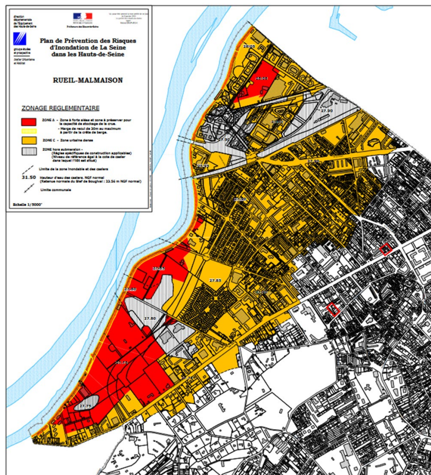
Figure 47 : Extrait du PPRI des Hauts de Seine
