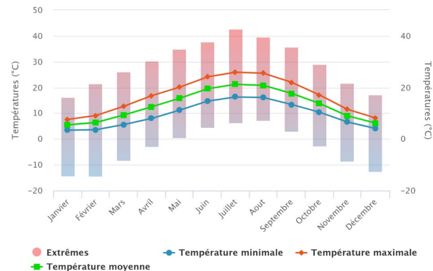
Figure 1 : Variation de la température sur l'année (période du 01/01/2000 au 31/12/2023)
